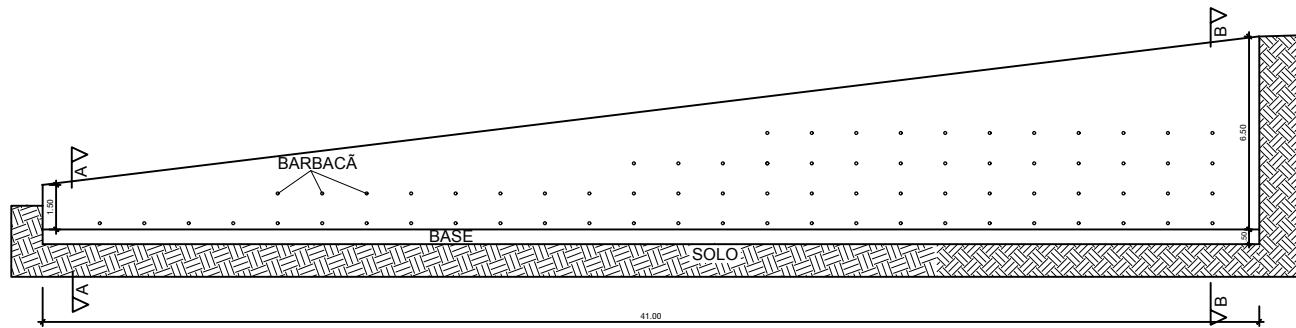
MURO 05 ESC: 1:75
