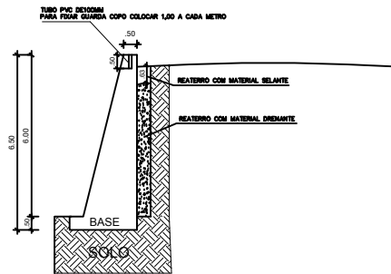
SEÇÃO BB 4,89 M2 ESC: 1:75
